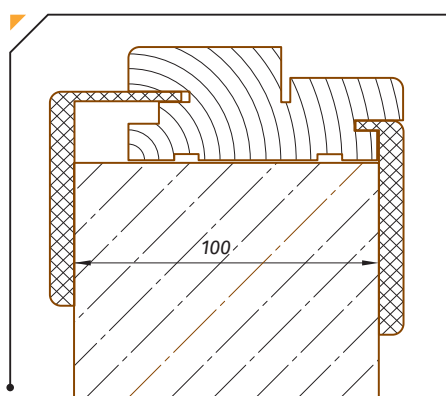
Схема збирання дверного короба з лиштвою
