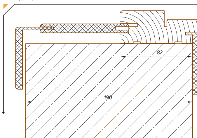
Схема збирання дверного короба з добірною планкою та лиштвою
