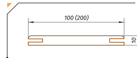
Добірна телескопічна планка
