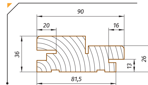
Дверний короб компланарний
